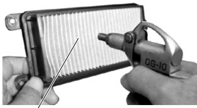
Elemento filtrante
